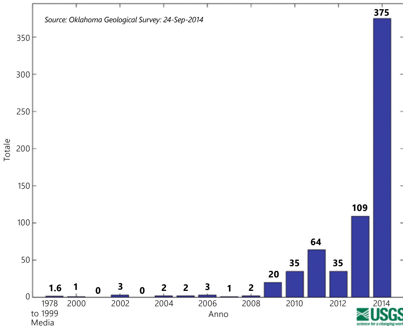
Il grafico del numero totale dei terremoti di magnitudo \geq 3 sulla scala Richter in Oklahoma nel 1978-2014
