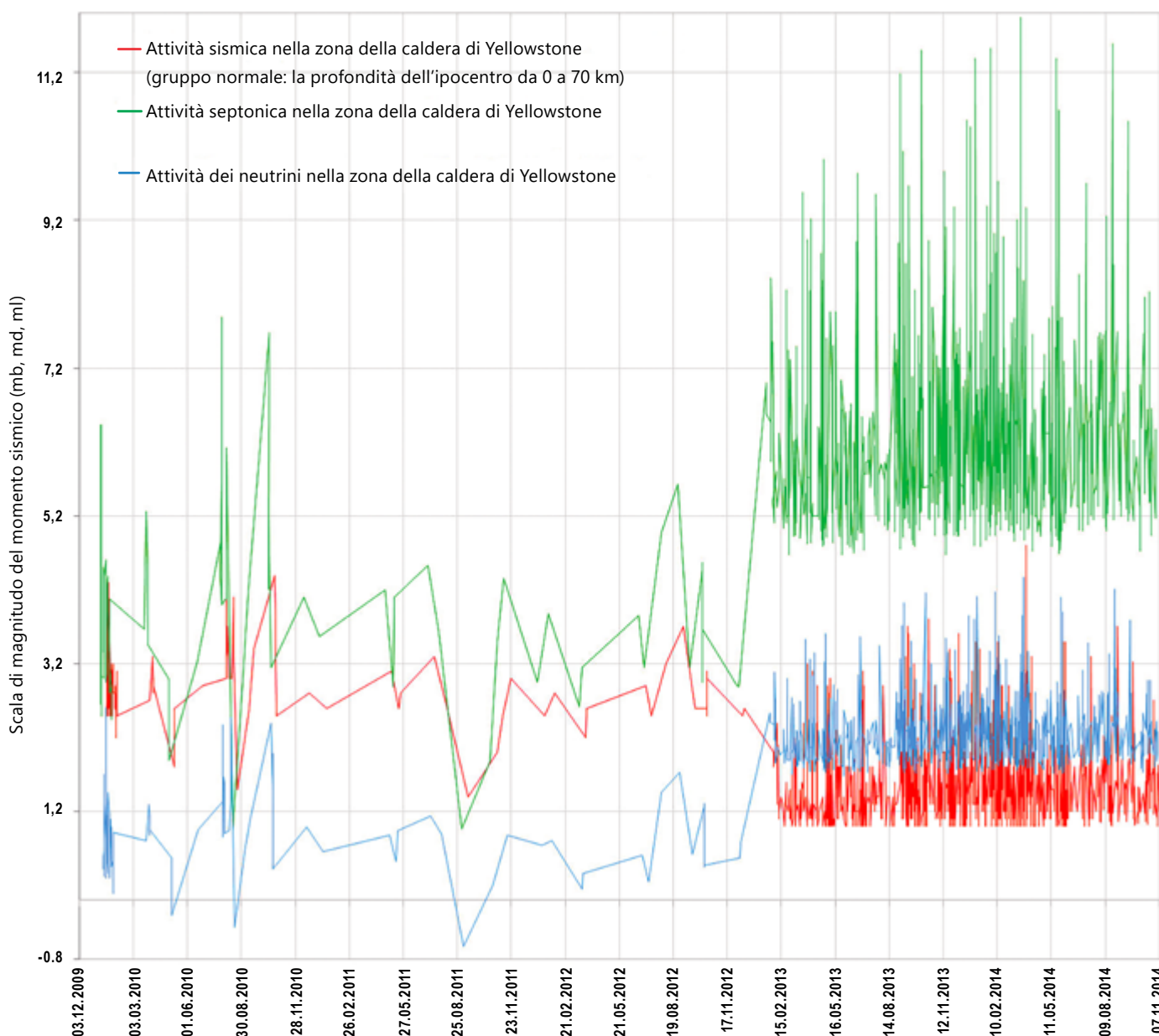
Attività sismica septonica e neutrina nella zona della caldera di Yellowstone (USA) nel 2010-2014 Grafico N° 14
