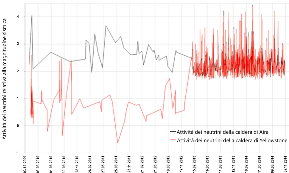
Attività septonica nella zona della caldera di Aira (Giappone) e nella zona della caldera di Yellowstone (USA) nel 2010-2014 Grafico N° 16
