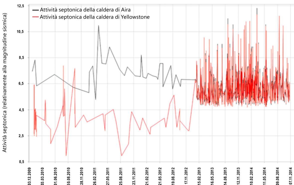
Attività septonica nella zona della caldera di Aira (Giappone) e nella zona della caldera di Yellowstone (USA) nel 2010-2014 Grafico N° 16
